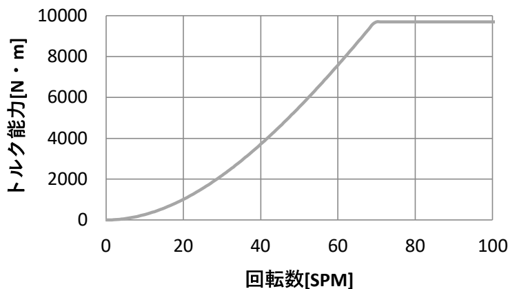
仕事能力線図
