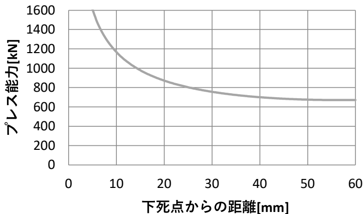
トルク能力線図(120mmSt)
