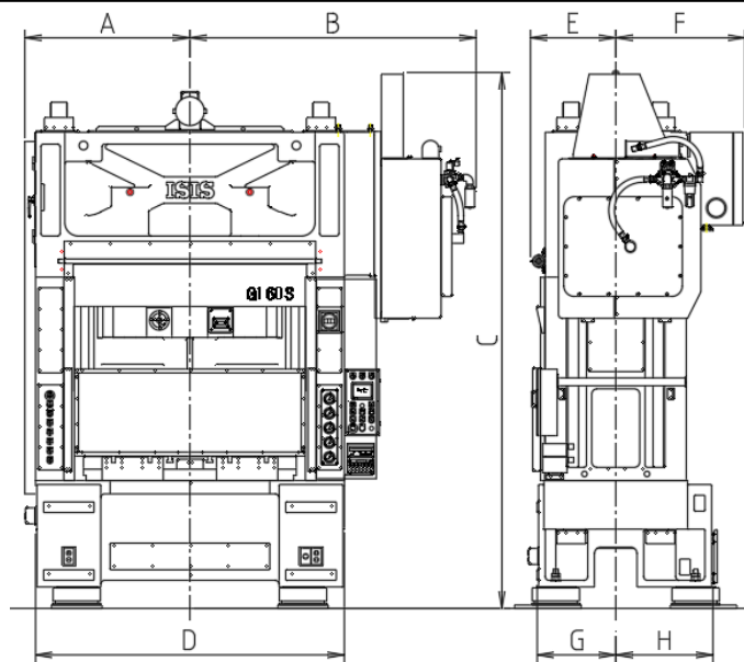
外形寸法図
