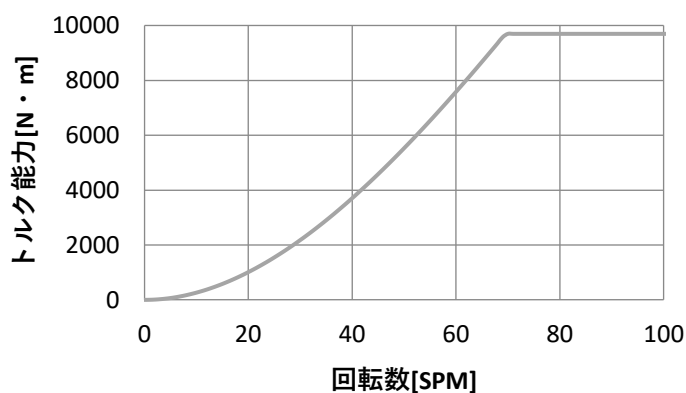
仕事能力線図
