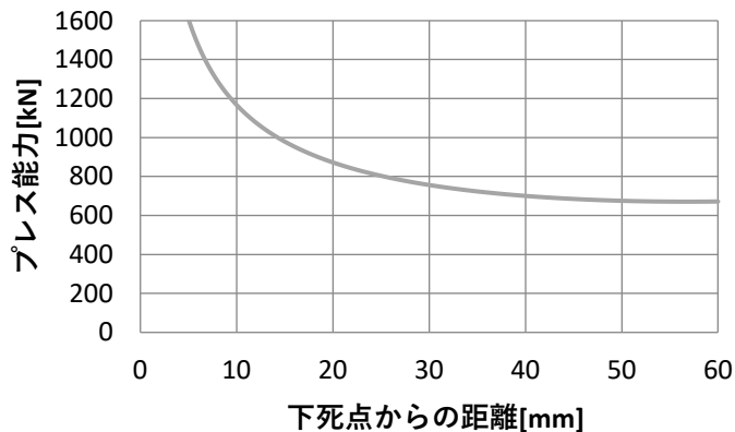
トルク能力線図(120mmSt)
